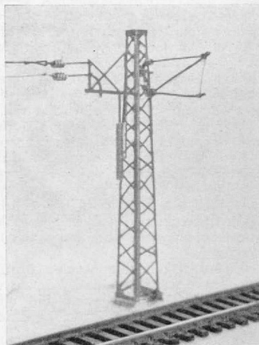
Abb. 10. Fahrdrabtverspannung bei Weichen ohne Überschneidung.
