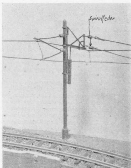
Abb. 7 und 8. Entwurf und H0-Ausführung eines Abspannmastes.
