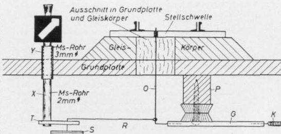
↓ Abb. 2. Schnitt durch die Weiche mit Laternendrehvorrichtung.
