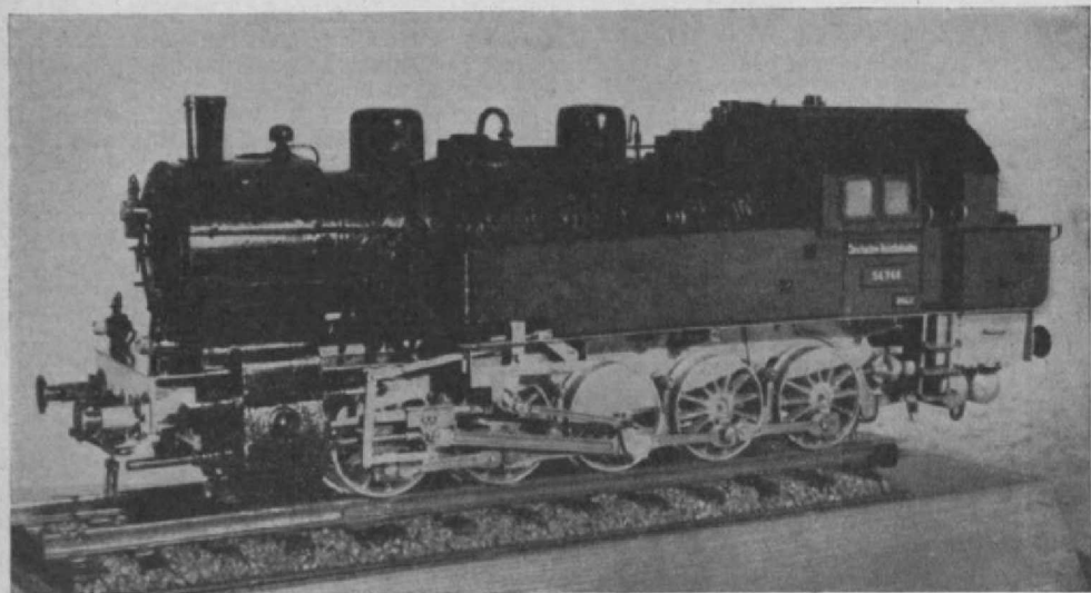
. . . baute Herr Ing. Böhme, Halberstadt, an diesem Modell einer E-Heißdampf-Güterzugtenderloks der Baureihe 94 (ehem. T 16 1 ) im Maßstab 1:27 (Spurweite 54 mm) Länge über Puffer 480 mm, größte Breite 122 mm, größte Höhe über S.O. 160 mm, Gewicht 4,27 kg.
