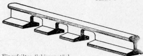
Eingeheiltes Schienenstück
