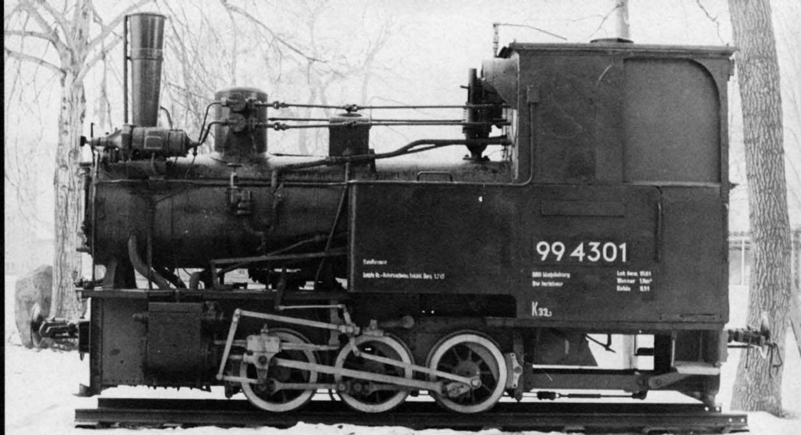
Bild 1: Die großen Überhänge vorn und hinten, der geringe Kuppelraddurchmesser von 600 mm und die bescheidene Bremsausrüstung erklären die auf 15 km/h festgesetzte Höchstgeschwindigkeit. Die Züge zum Dampfdom auf der Heizerseite sind mit Kardangelen versehen.
