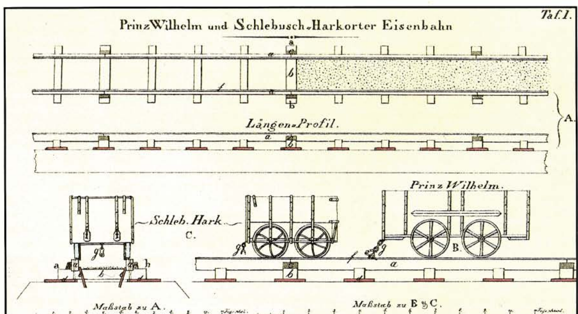
Bild 6: Gleis und Wagen der mit Pferden betriebenen Prinz-Wilhelm- und Schlebusch-Harkorter Eisenbahn aus Friedrich Harkorts Schrift "Die Eisenbahn von Minden nach Cöln" von 1833. Stadtarchiv Hagen
