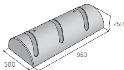
Stojan na kolo SK 2 – 3
