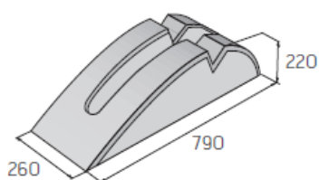
Stojan na kolo SK 1 – 1
