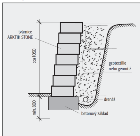
Schematický náčrt uložení tvárnice ARKTIK STONE
