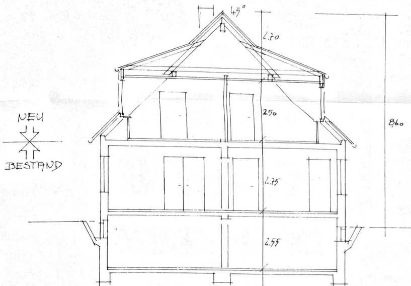
SCHNITT A-A
