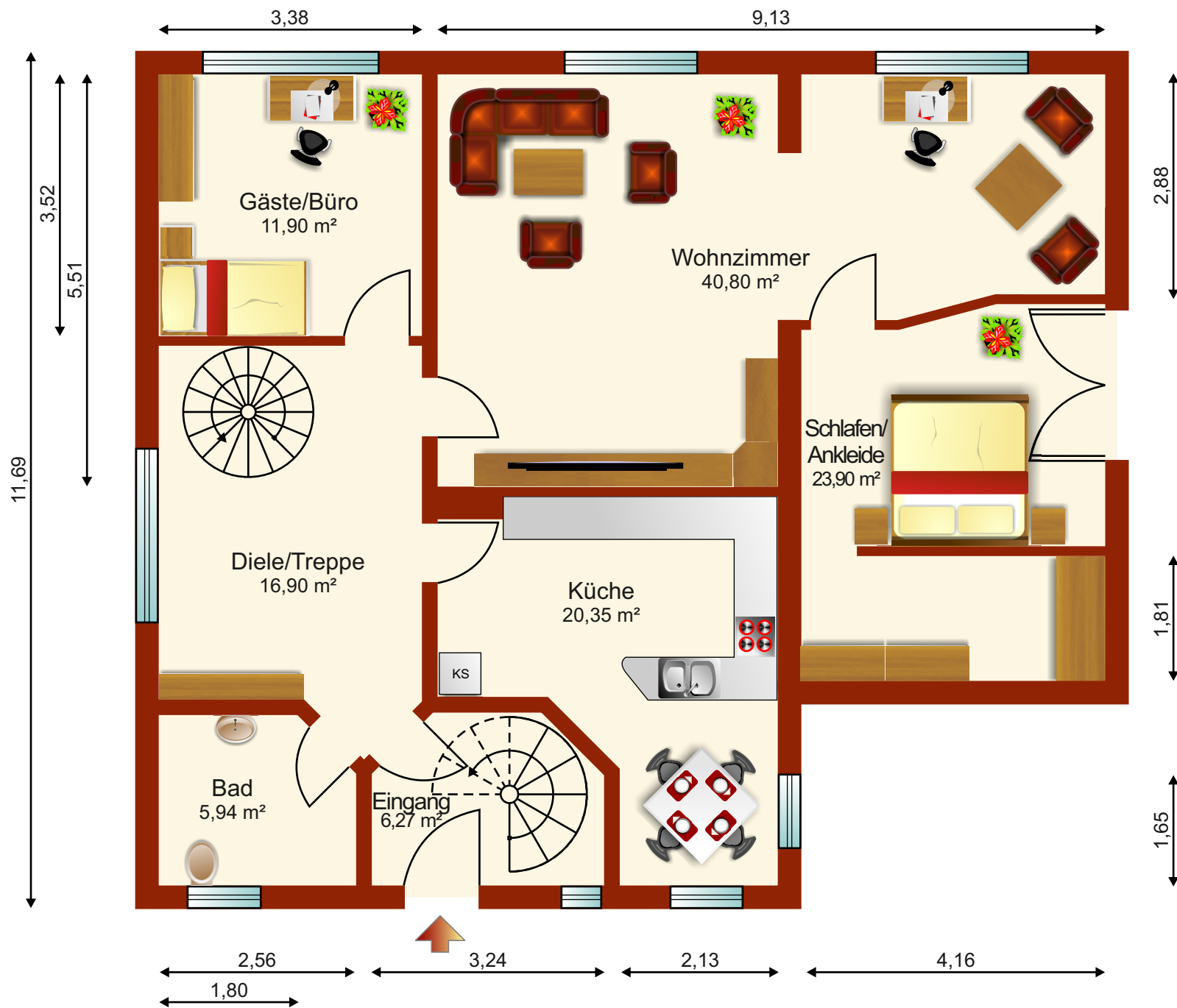
Erdgeschoss
