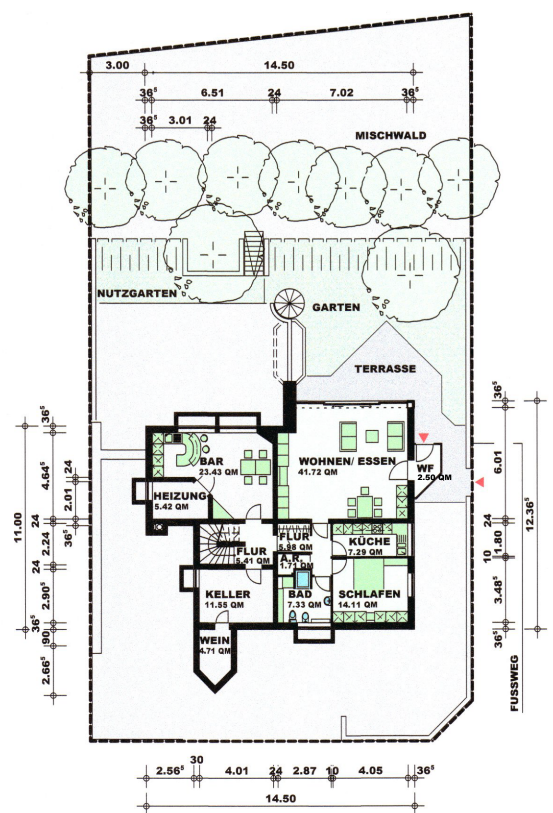
UNTERGESCHOSS M 1: 200 EINLIEGERWOHNUNG CA. 80,64 QM
