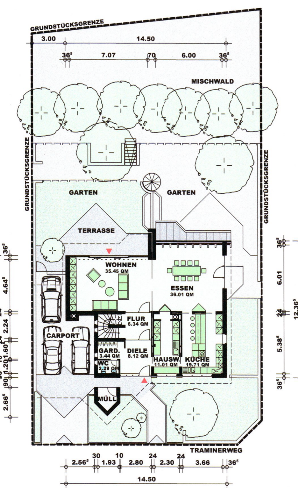
ERDGESCHOSS M 1: 200 HAUPTWOHNUNG CA. 122,37 QM
