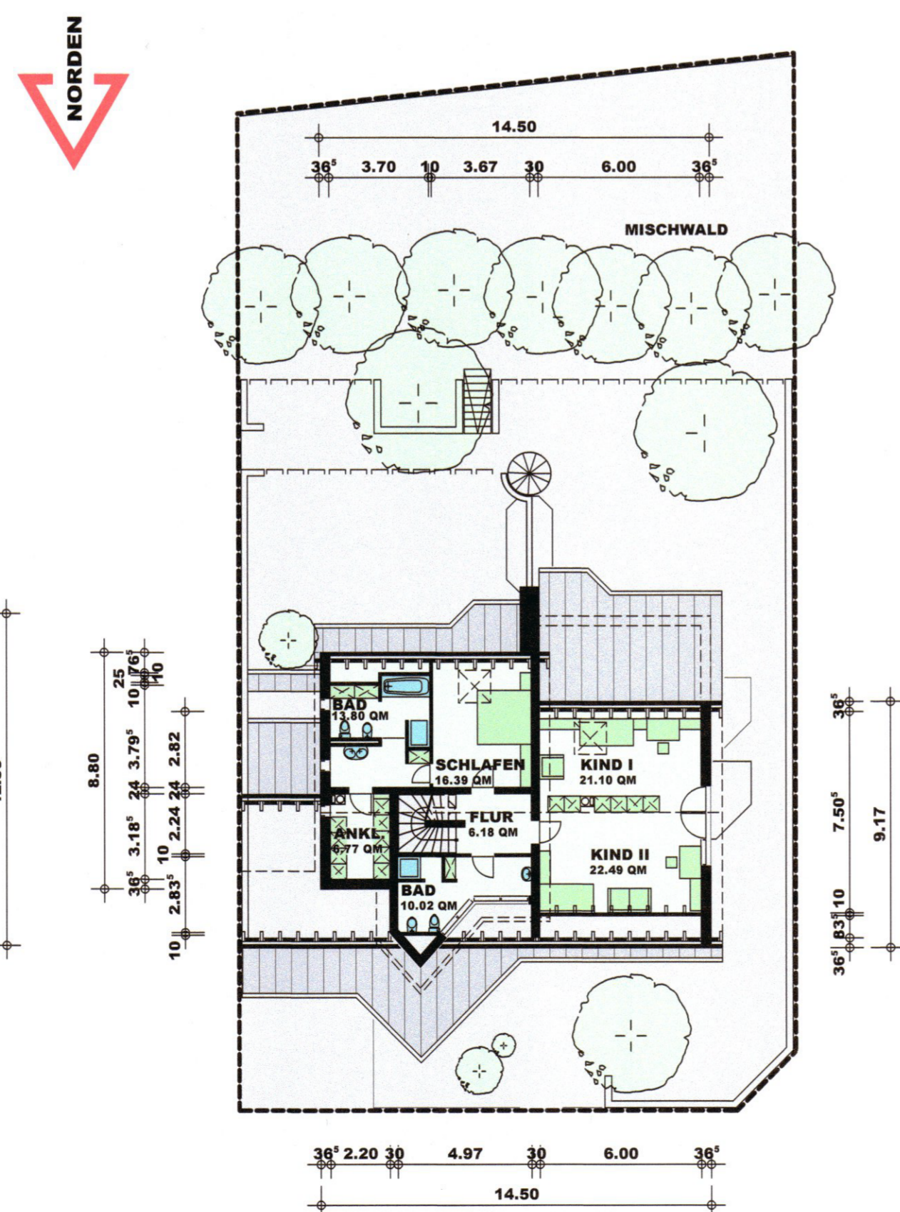
OBERGESCHOSS M 1: 200 HAUPTWOHNUNG CA. 95,75 QM
