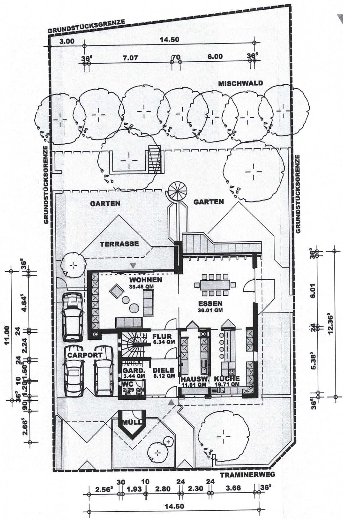
ERDGESCHOSS M 1: 200 HAUPTWOHNUNG CA. 122,37 QM
