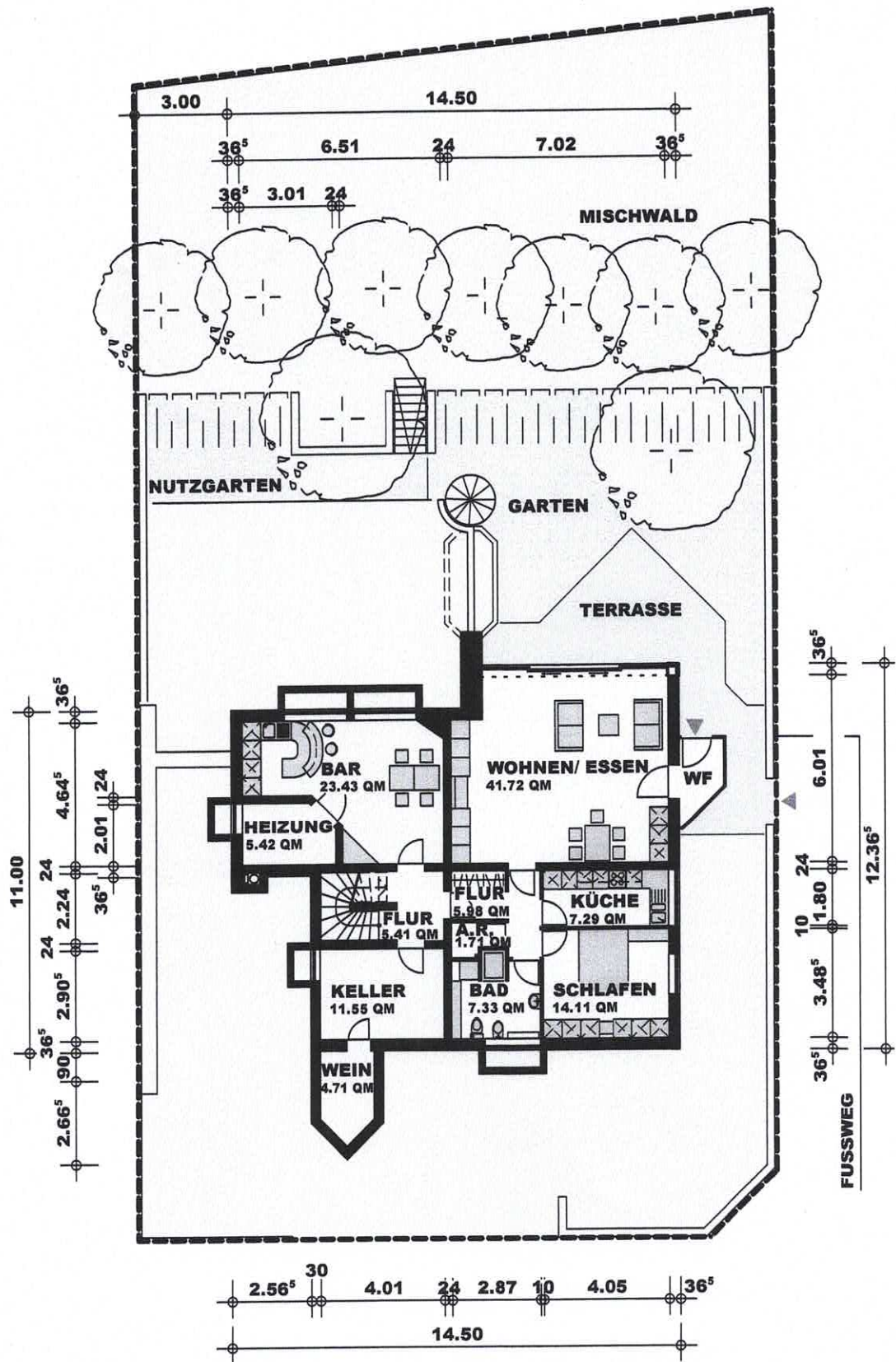
UNTERGESCHOSS M 1: 200 EINLIEGERWOHNUNG CA. 83.55 QM
