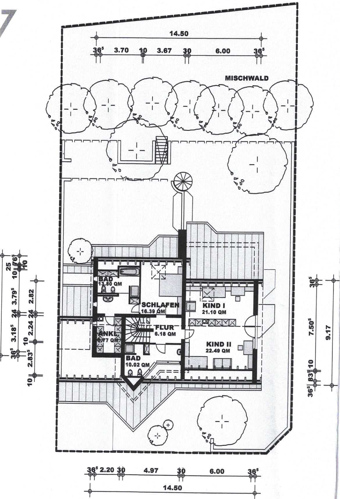
OBERGESCHOSS M 1: 200 HAUPTWOHNUNG CA. 96.75 QM
