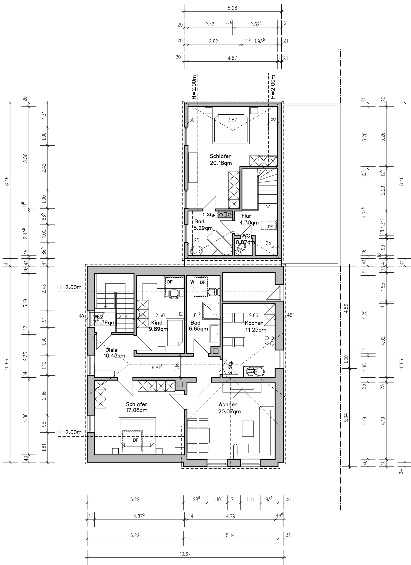
Dachgeschoss
