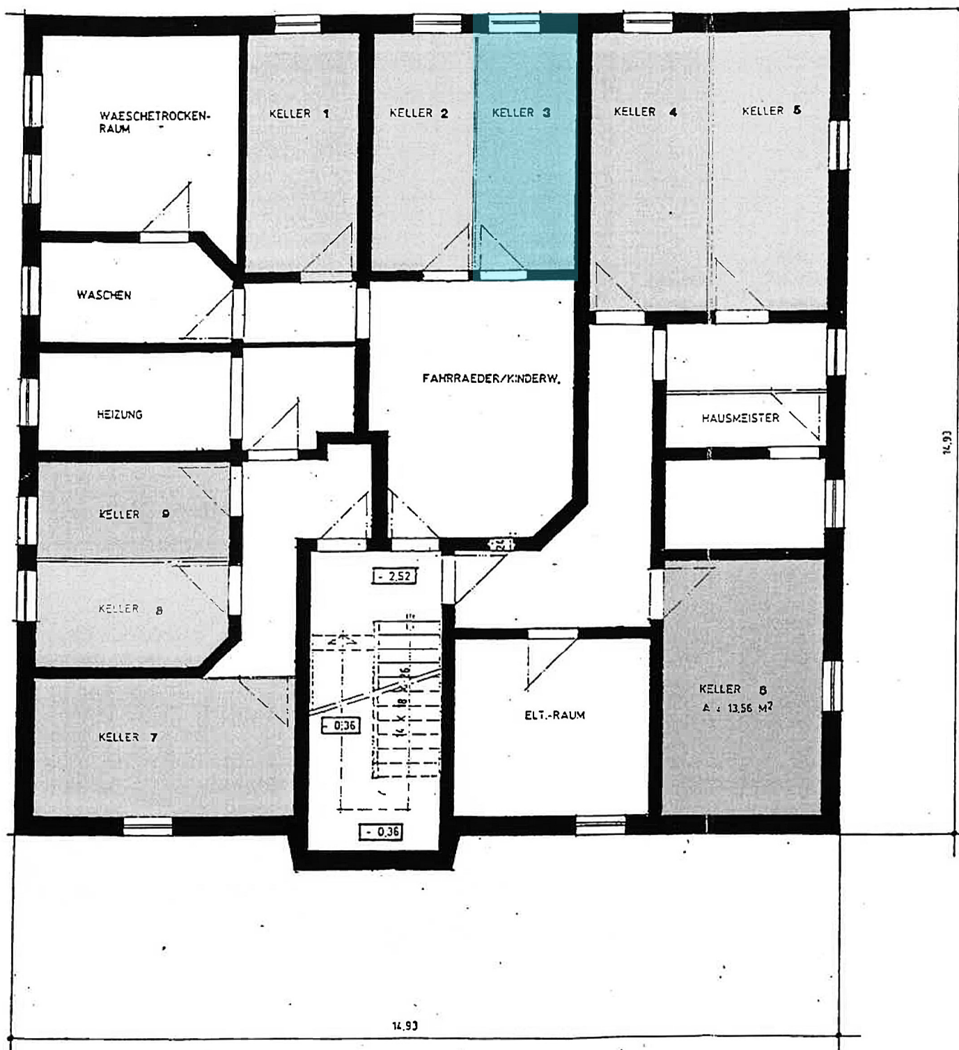
Grundriß Keller
