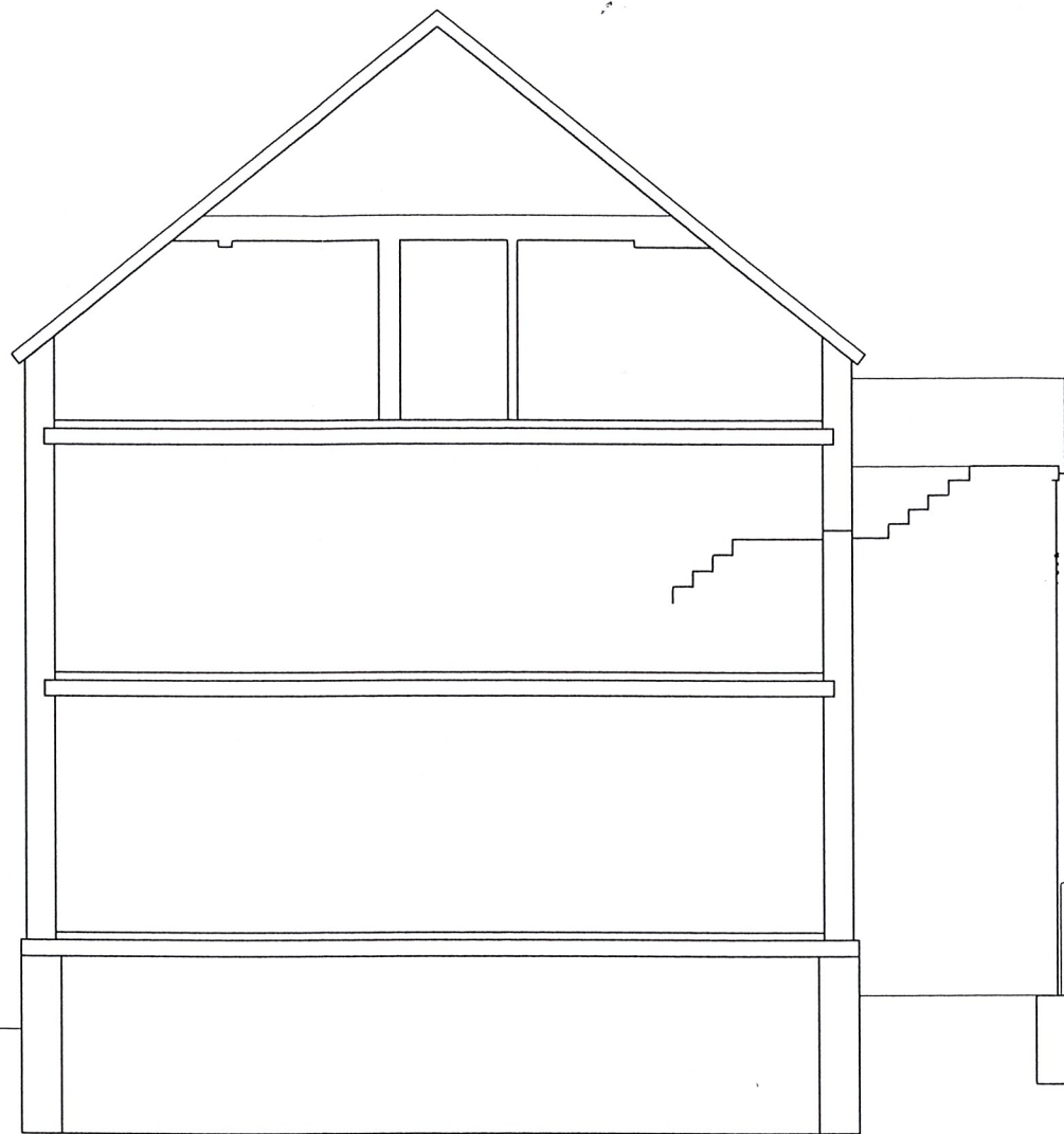
Schnitt vorhanden
