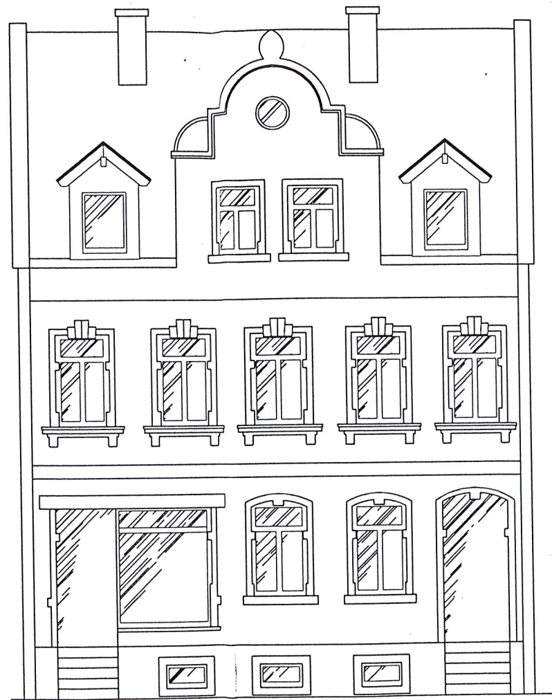
Ausicht Straßenseite
