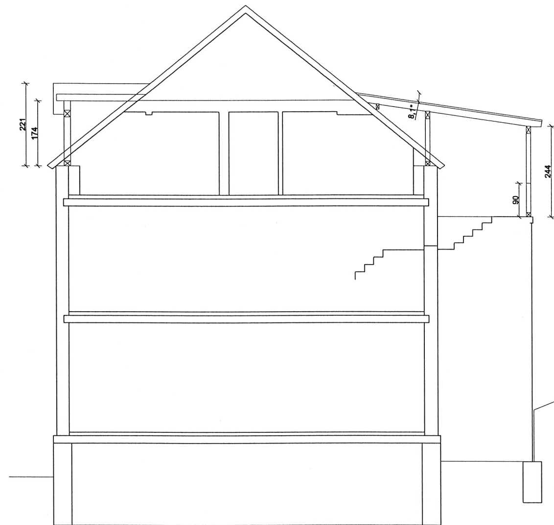
Schnitt Planung
