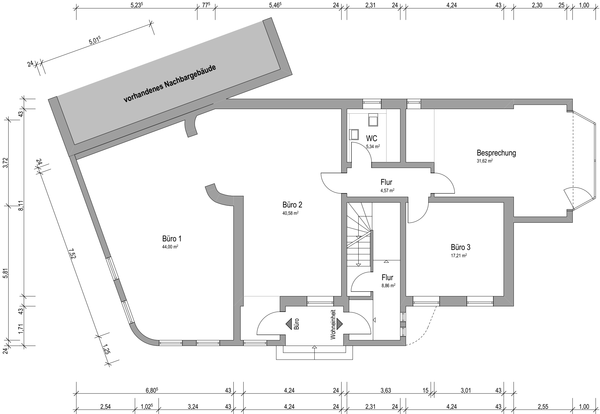
Erdgeschoss
