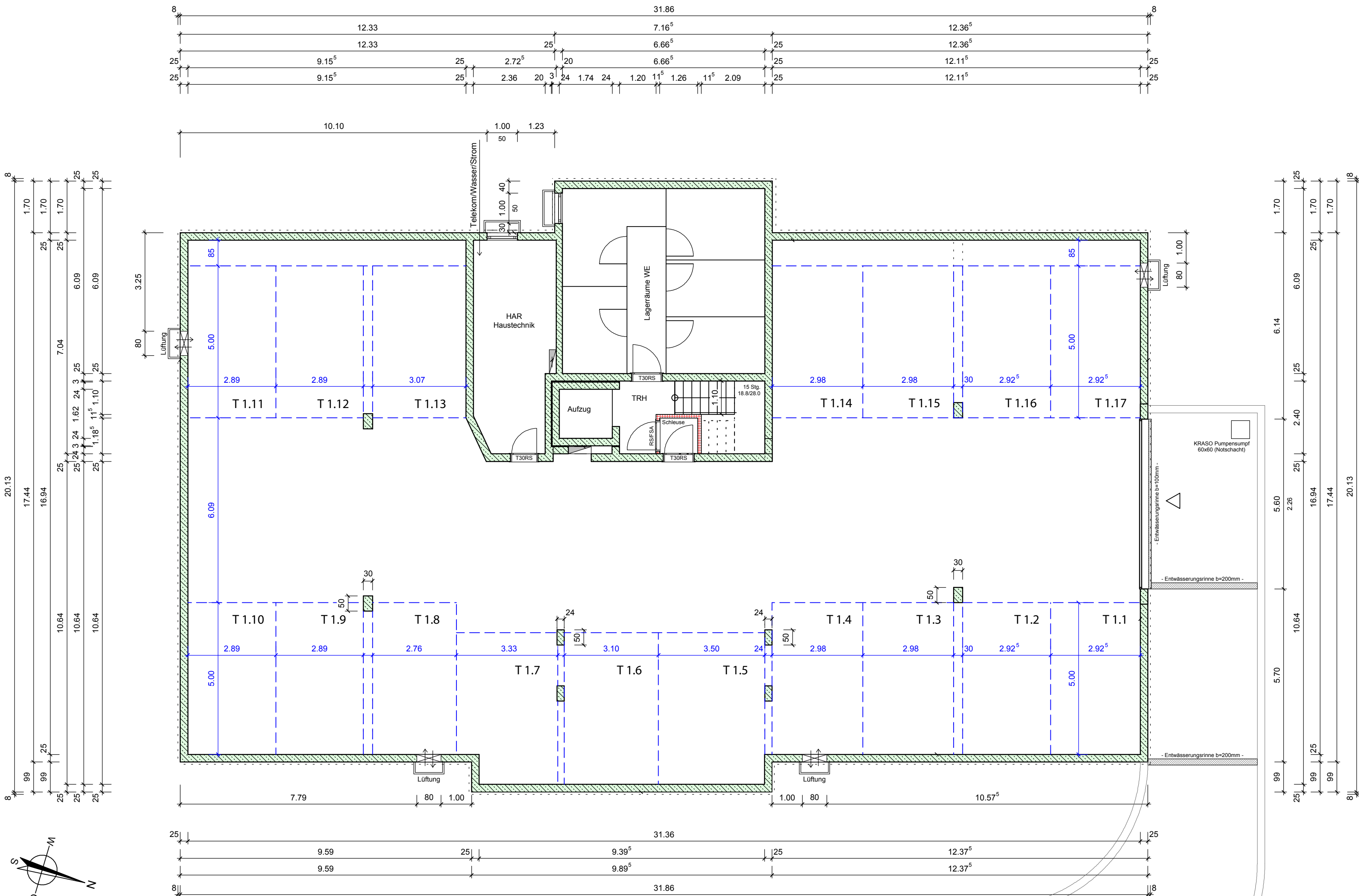
Untergeschoss
