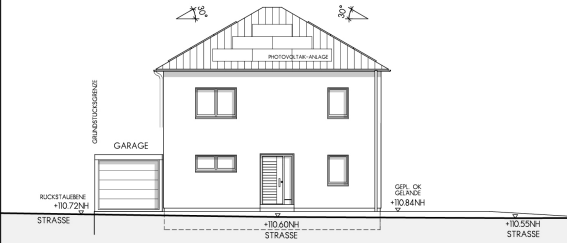
ANSICHT SUD
