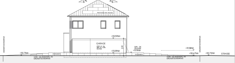
ANSICHT WEST
