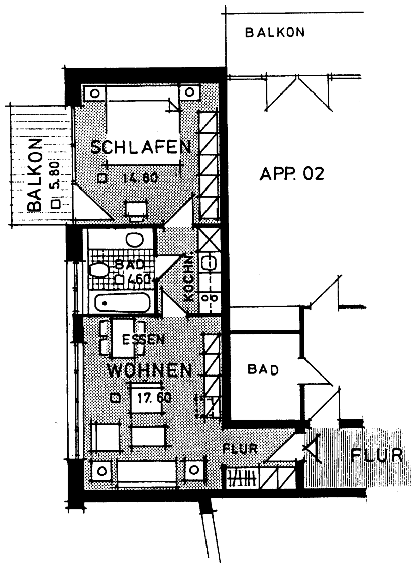
Grundriss Wohnung Nr. 1
