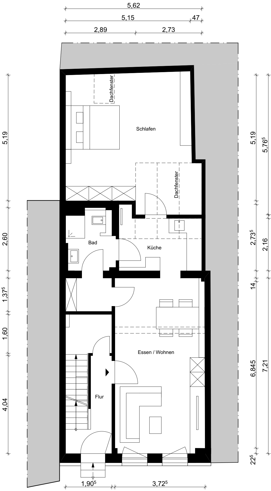
Erdgeschoss M. 1:75
