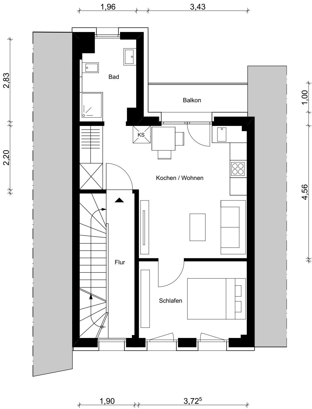
1.OG M. 1:75
