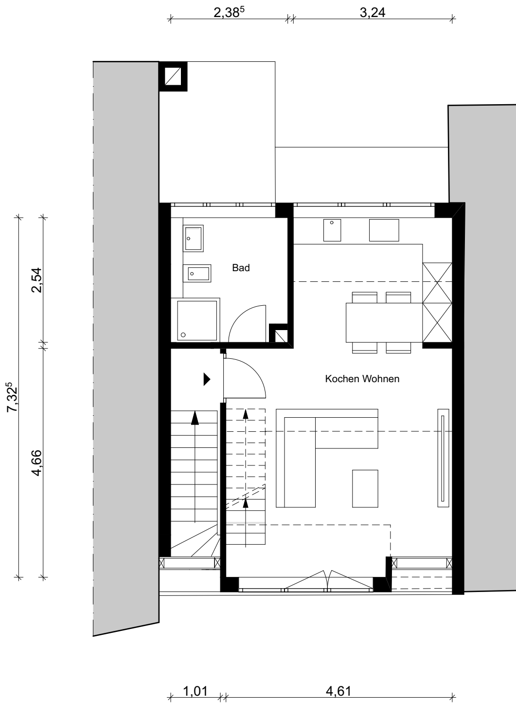
DG M. 1:75
