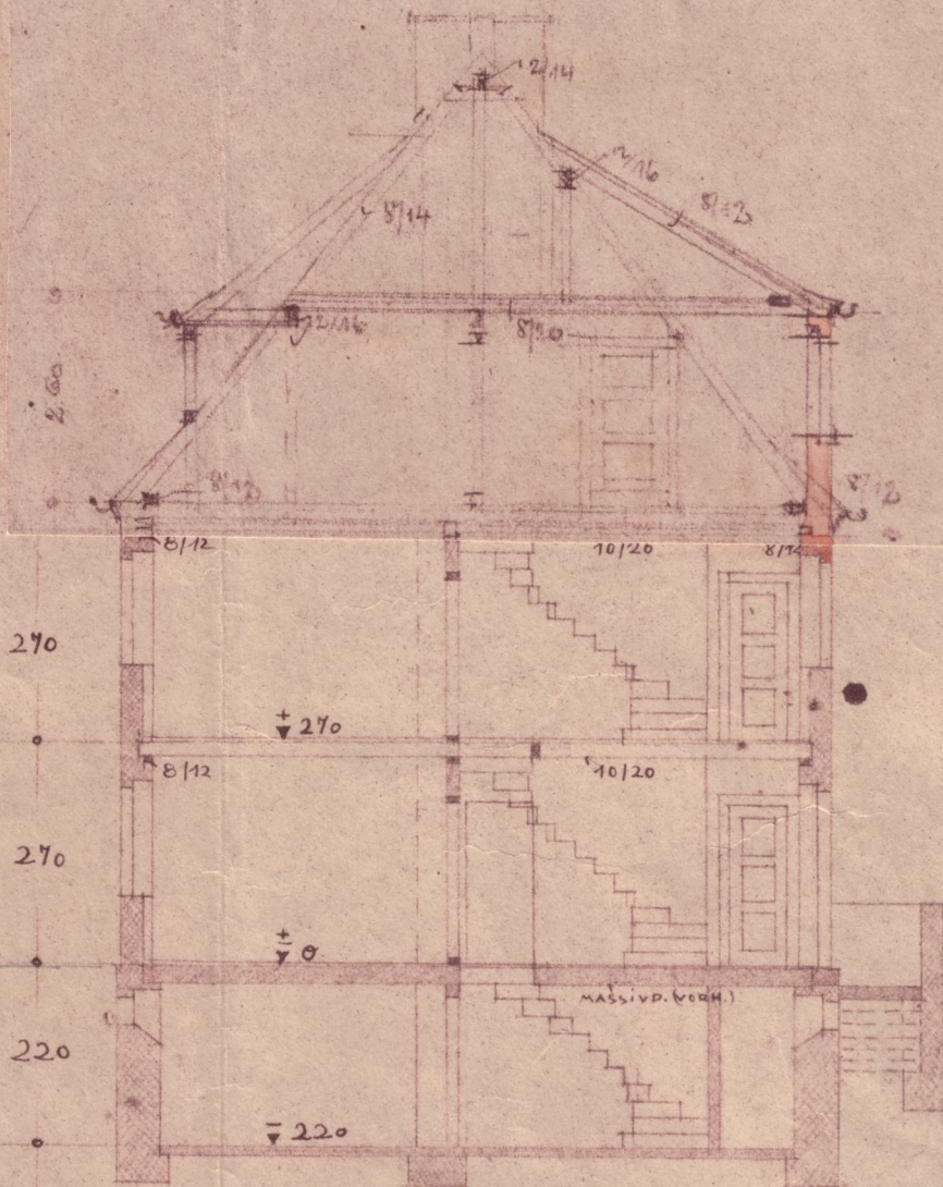
SCHNITT = C-D
