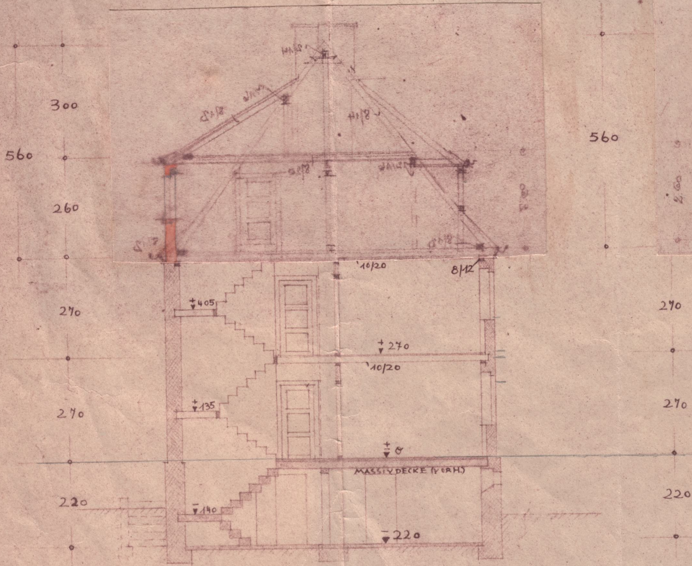
SCHNITT A-B
