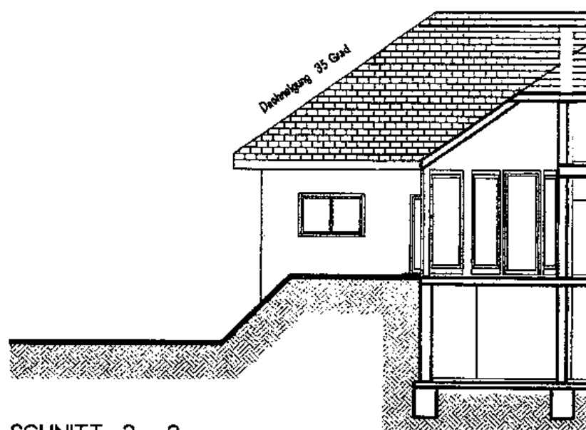
SCHNITT 3 - 3
