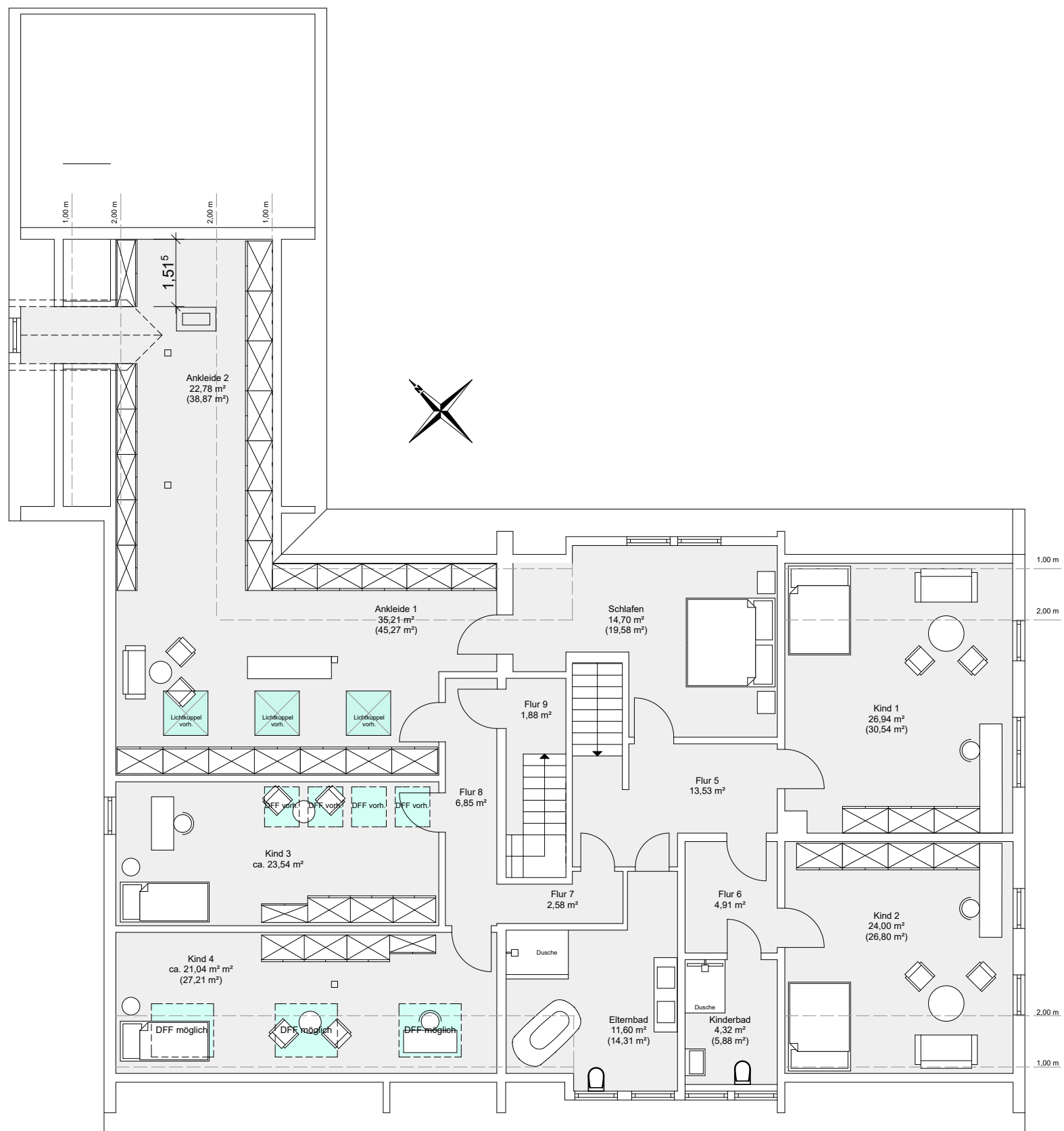
ObergeschossVariante 2 Lofraum: 2 weitere Kinderzimmer
