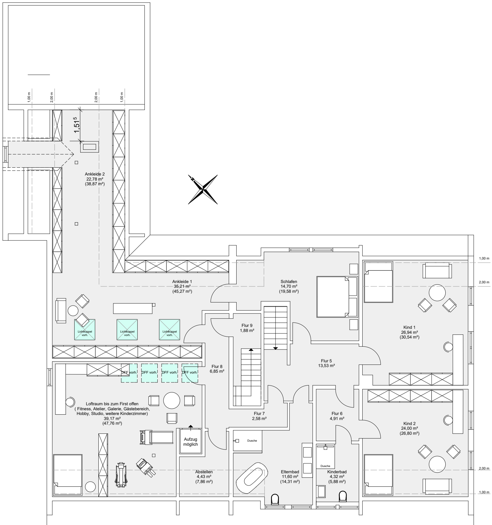
Obergeschoss Variante 1 Lofraum: Fitness/Atelier/Hobby/Gäste, etc.
