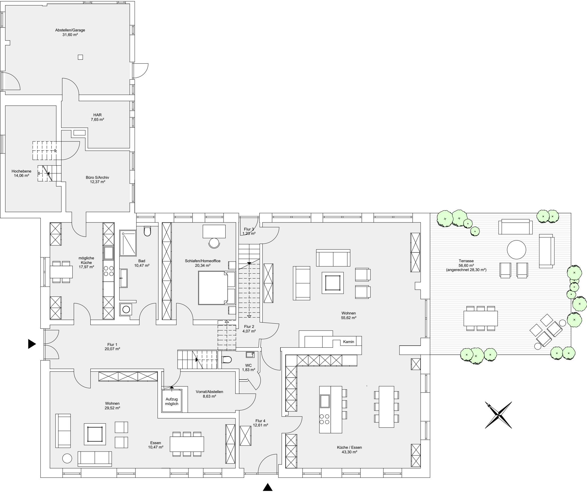
Erdgeschoss Variante 2: Einliegerwohnung
