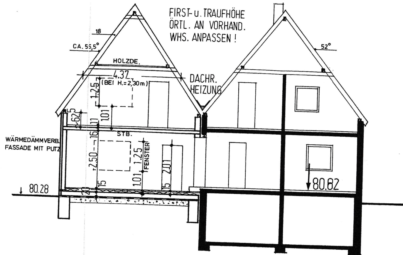
SCHNITT A-B
