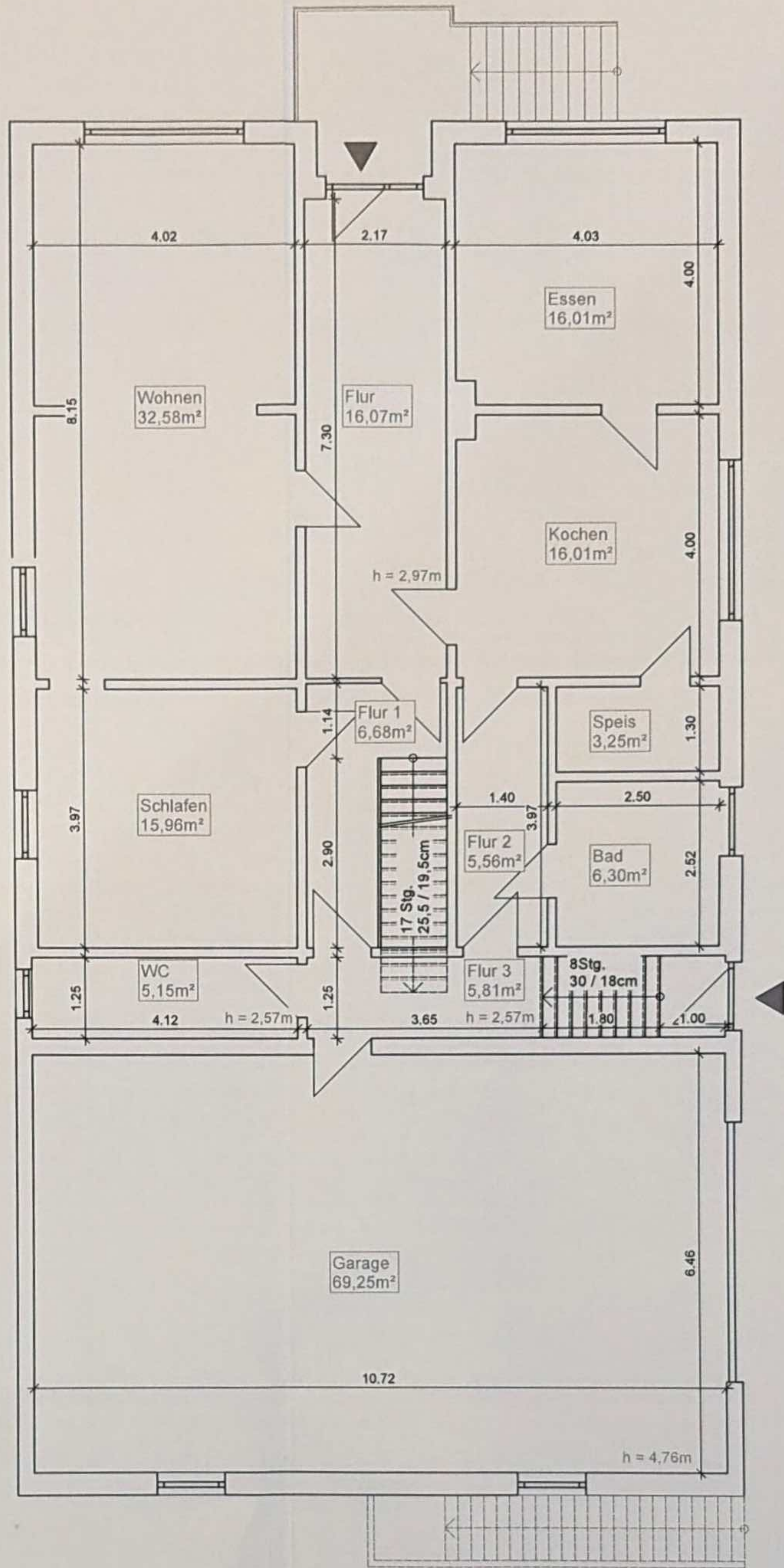
Grundriss Erdgeschoss
