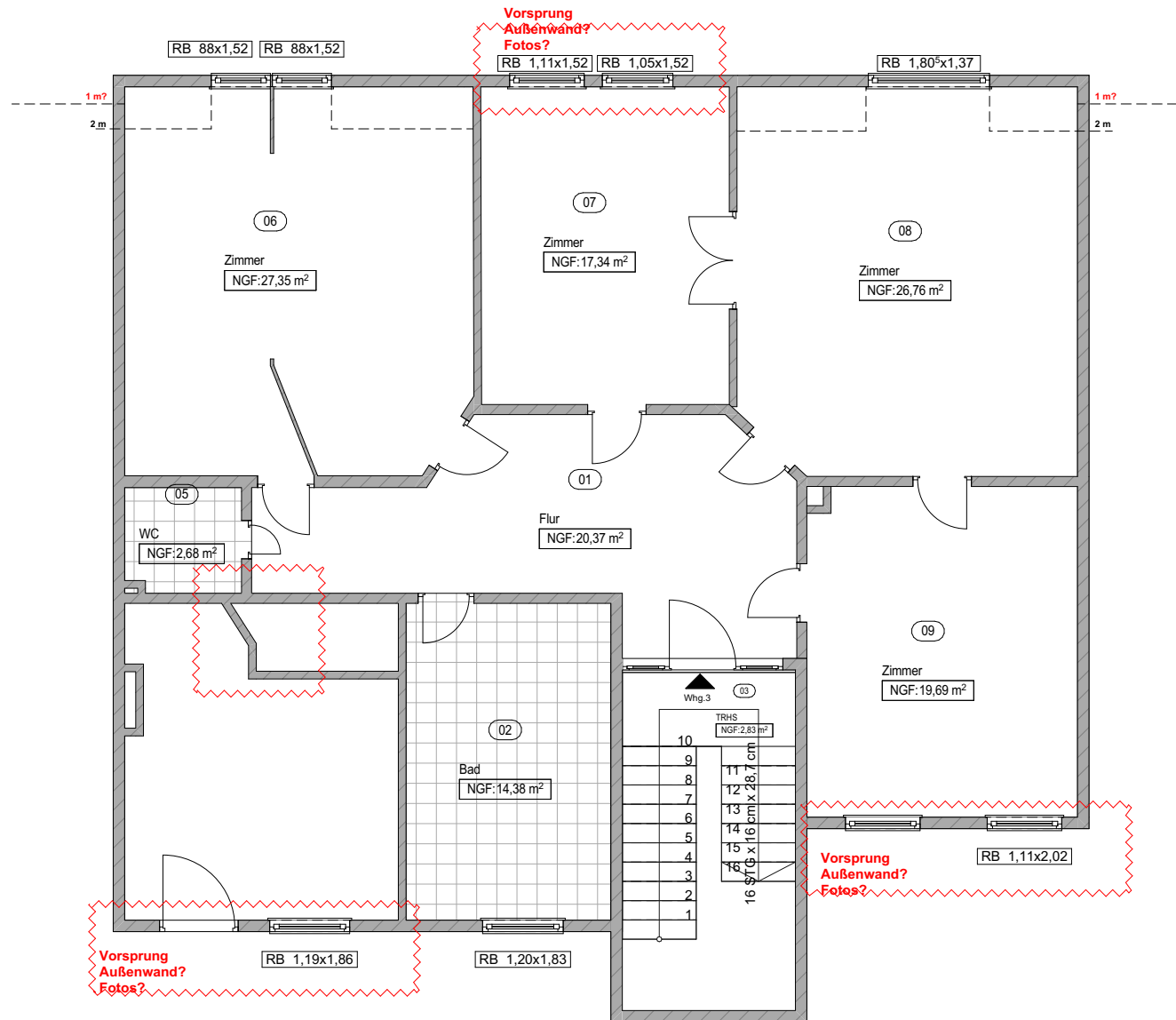
Grundriss 3. Obergeschoss Wohnung
