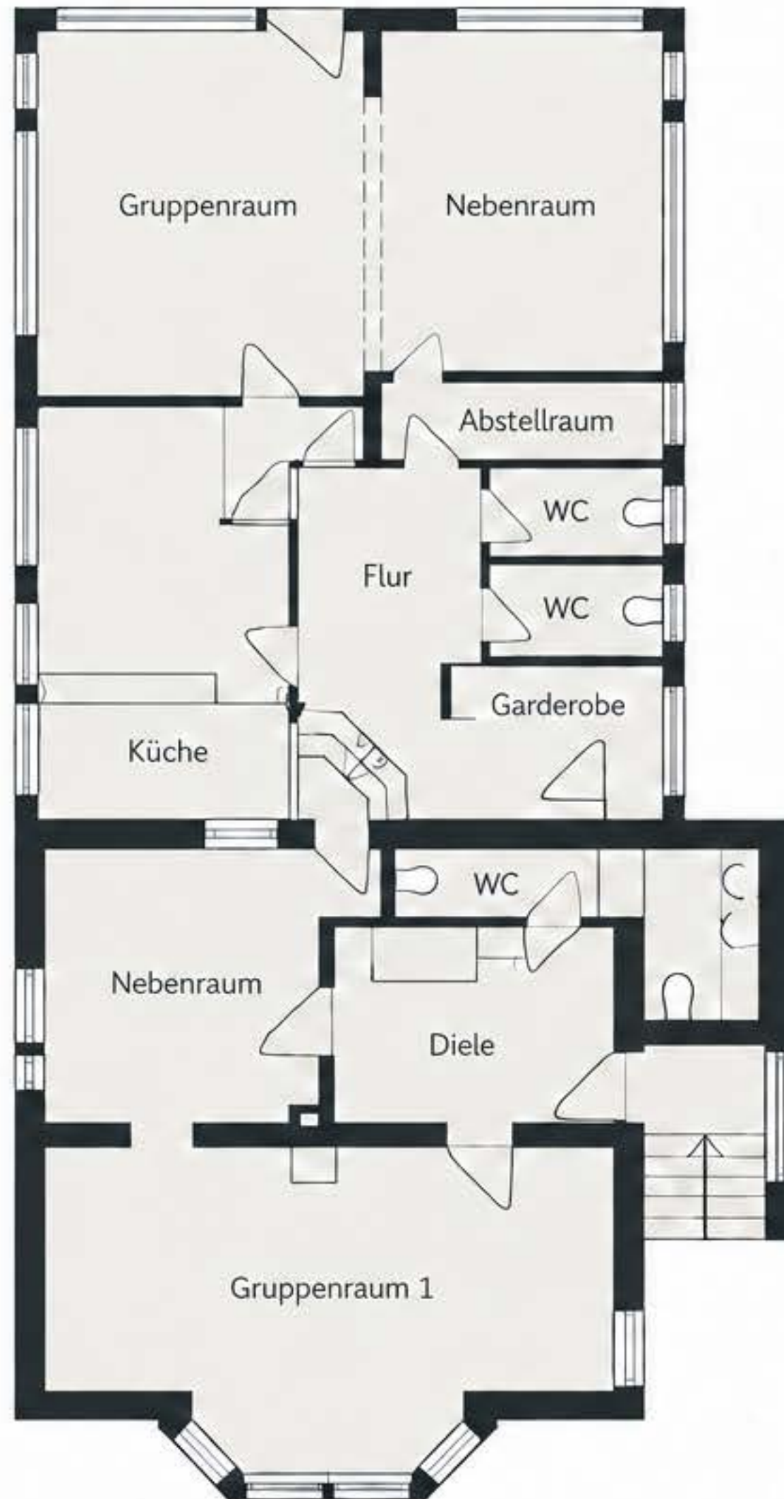
Erdgeschoss
