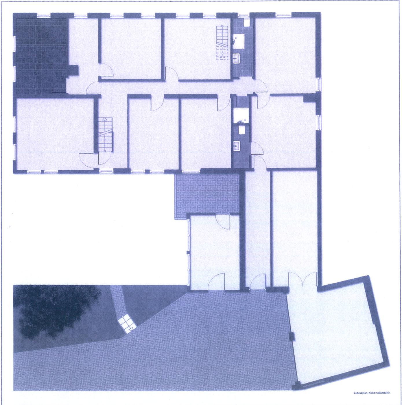
Obergeschoss
