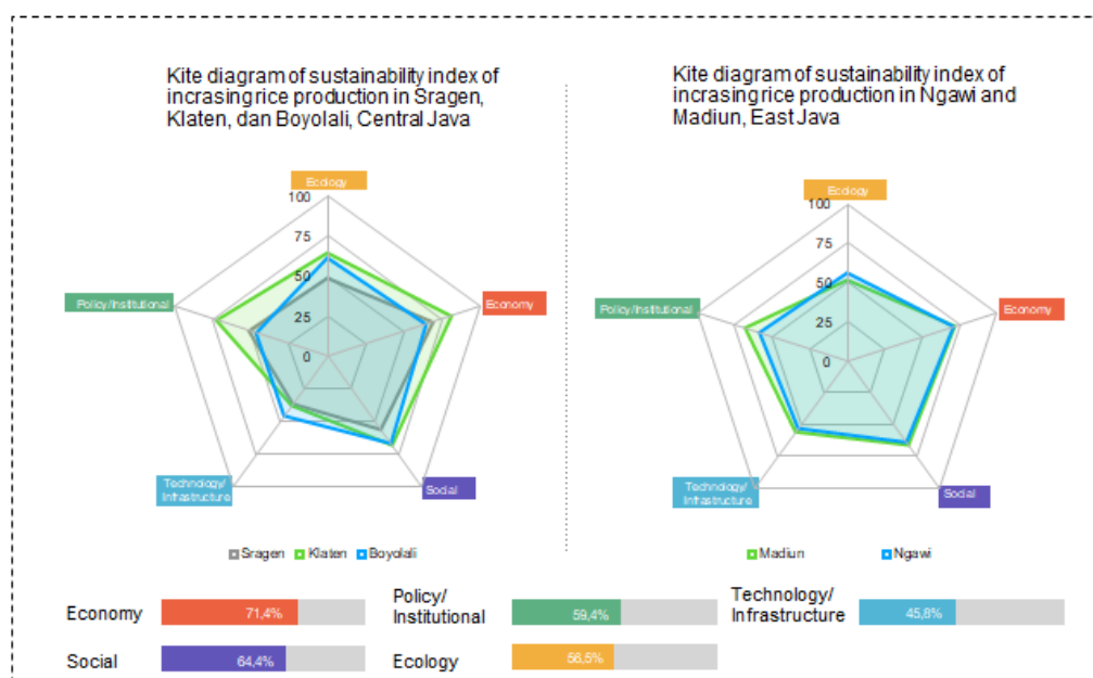
Gambar 2 Indeks Keberlanjutan Budidaya Padi di Sentra Produksi Padi
