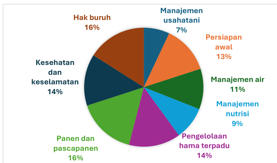
Gambar 3 Bobot SRP Indonesia untuk Standar Budidaya Padi Berkelanjutan
