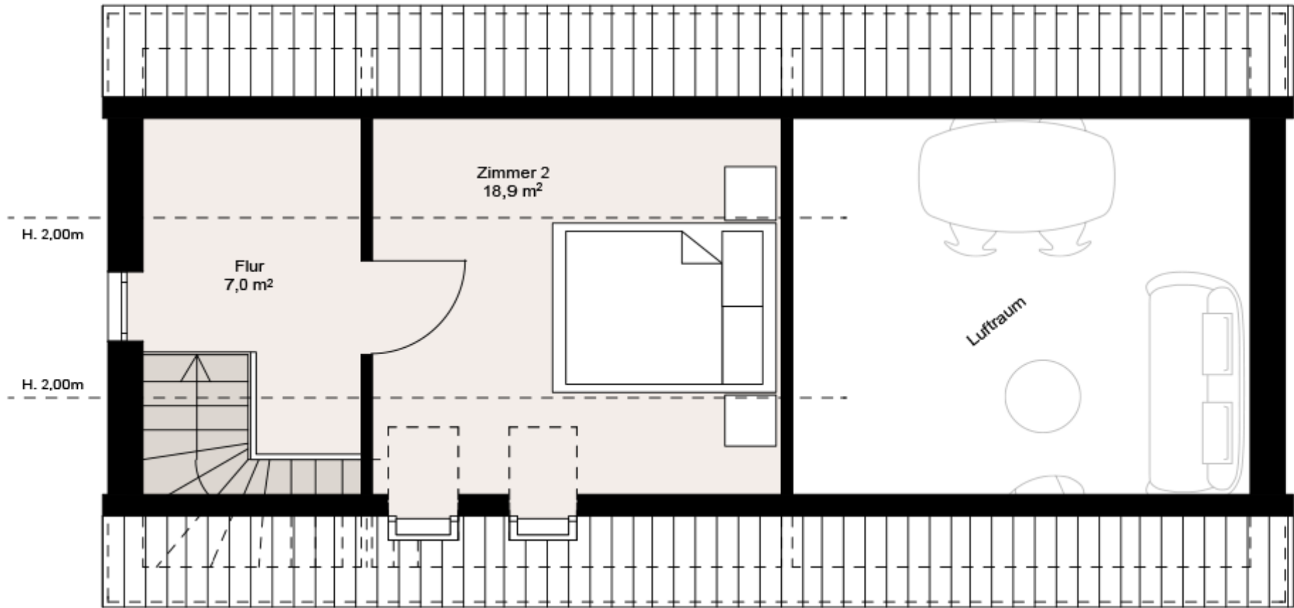
Grundriss OG
