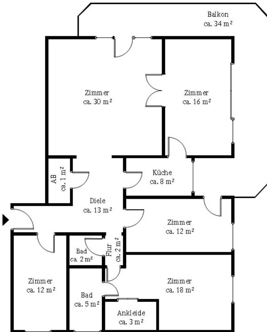
1. Obergeschoss
