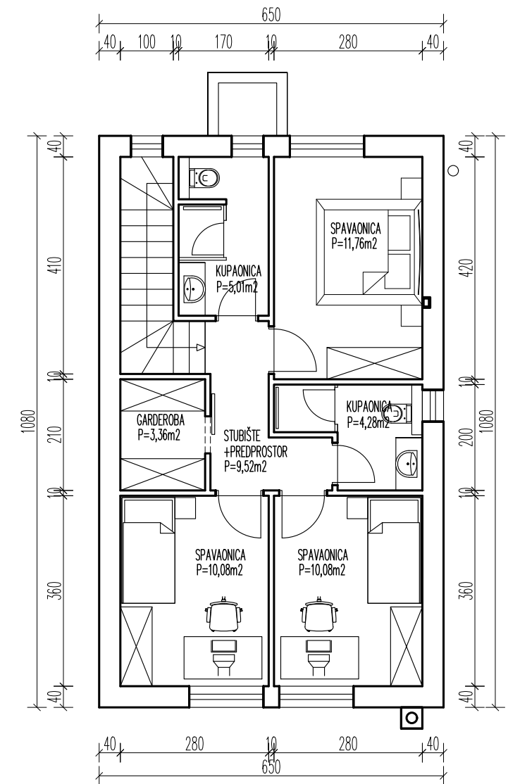
TLOCRT KATA
