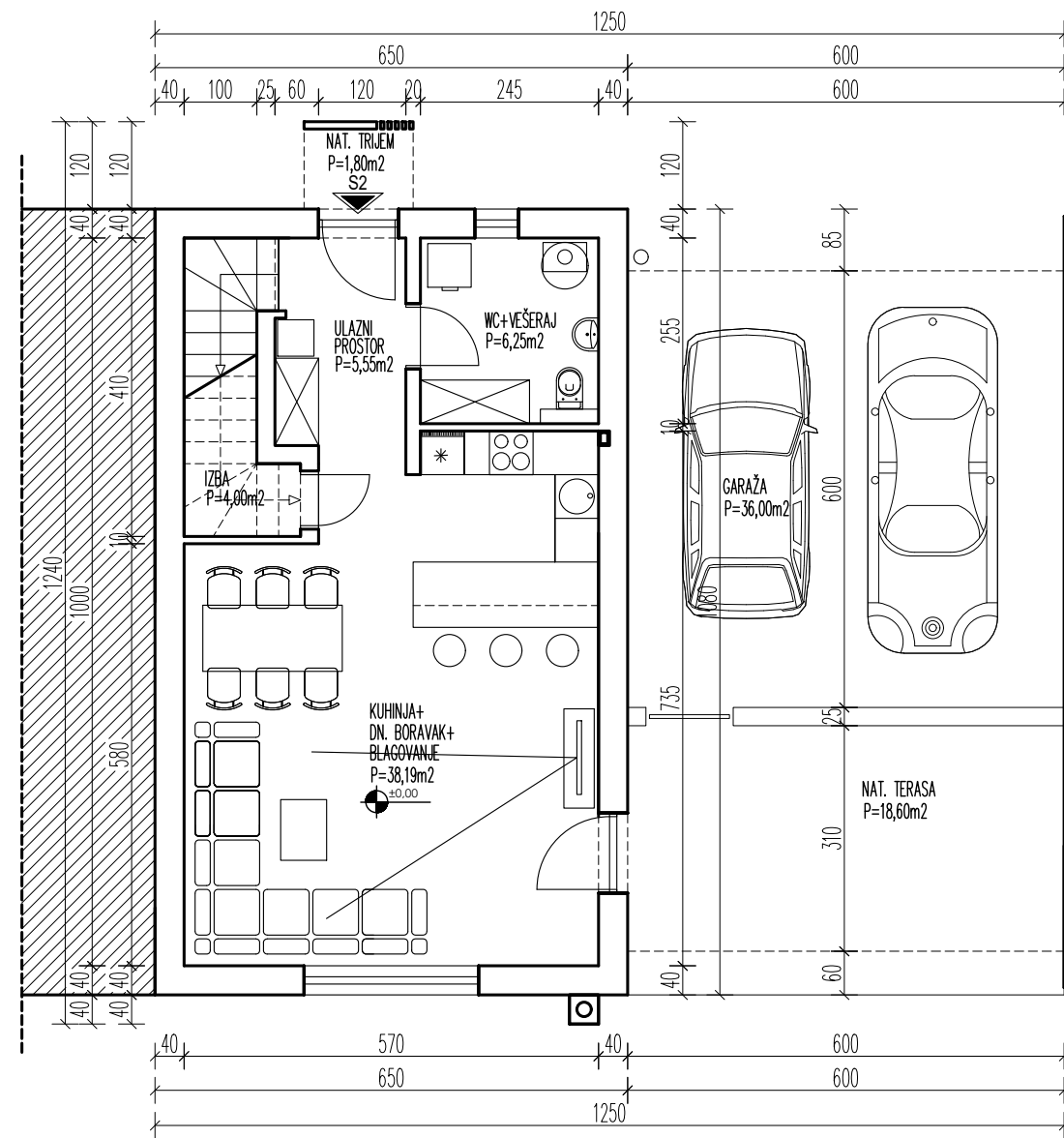
TLOCRT PRIZEMLJA
