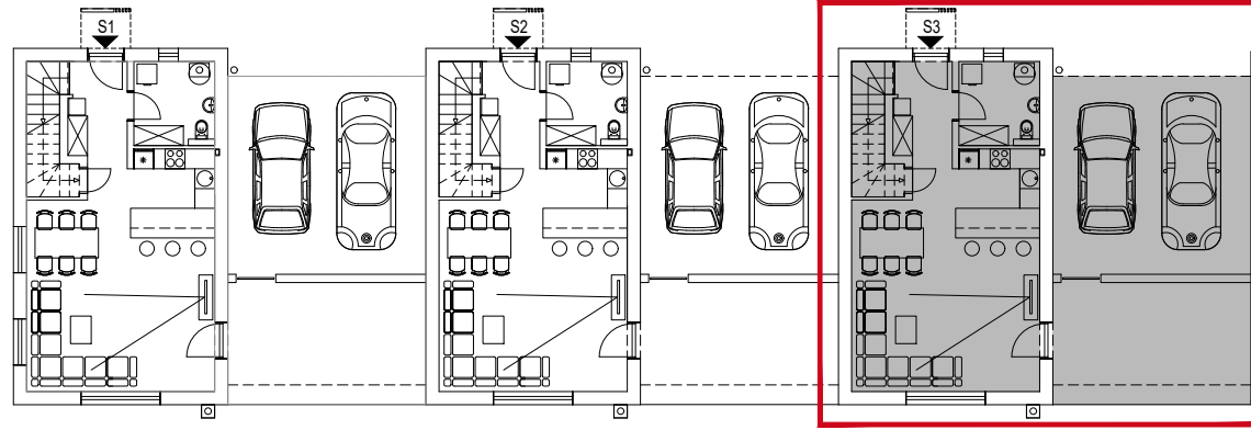
TLOCRT PRIZEMLJA
