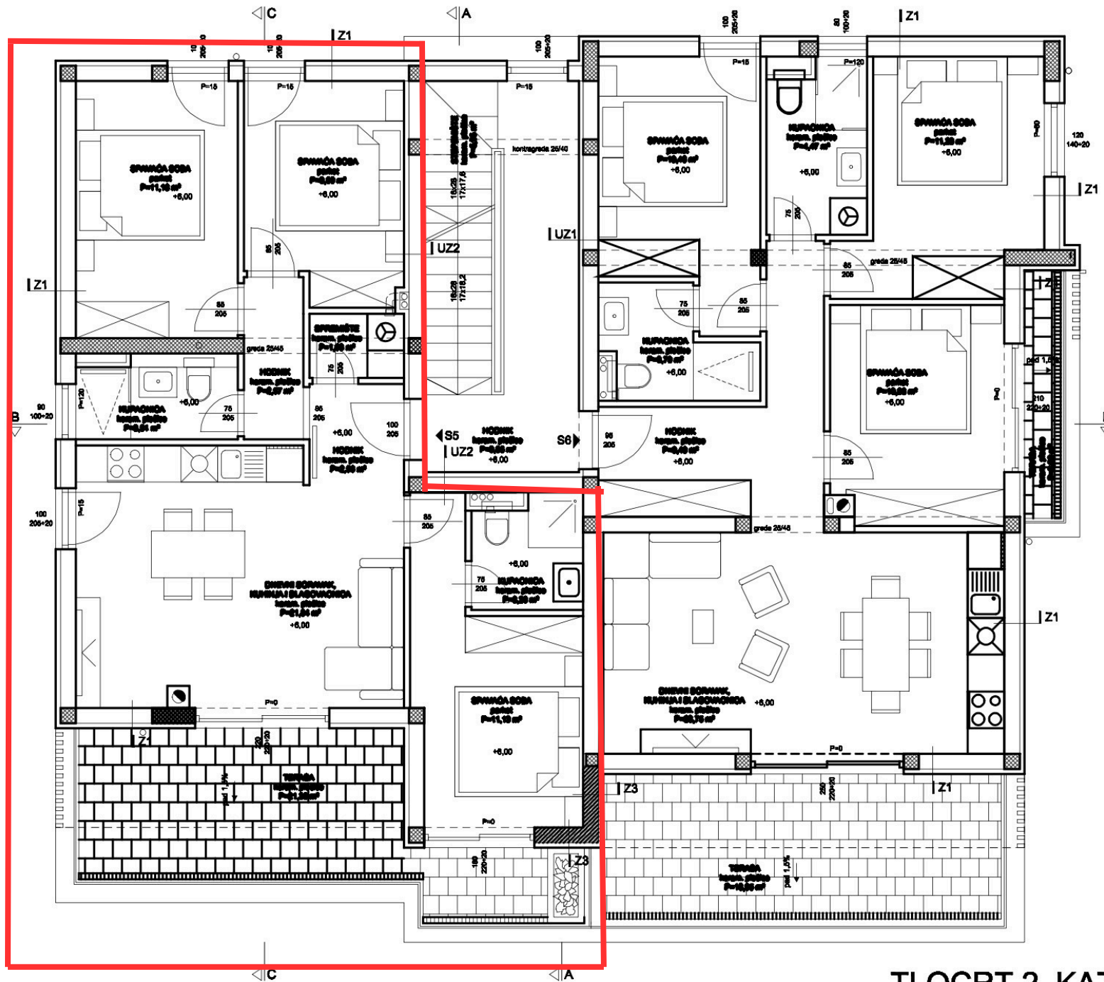
TLOCRT 2. KATA
