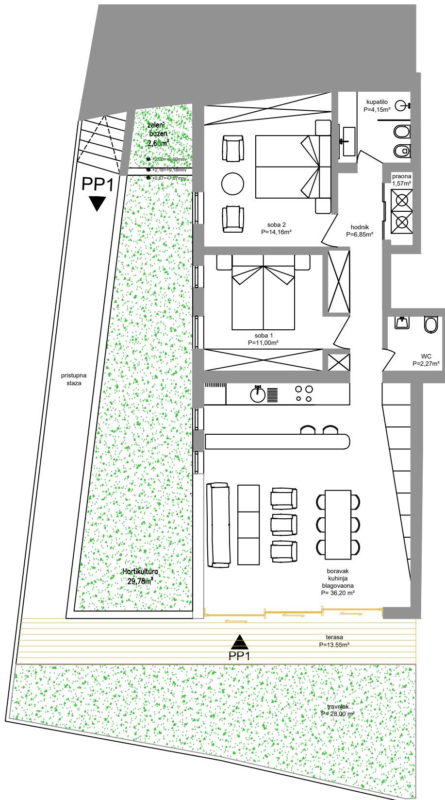
Layout stan PP1_nisko prizemlje
