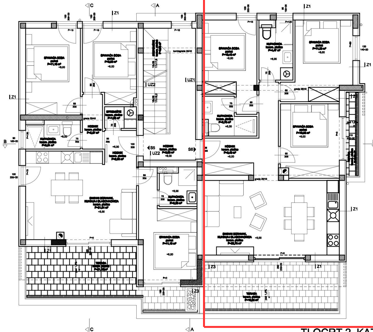
TLOCRT 2. KATA
