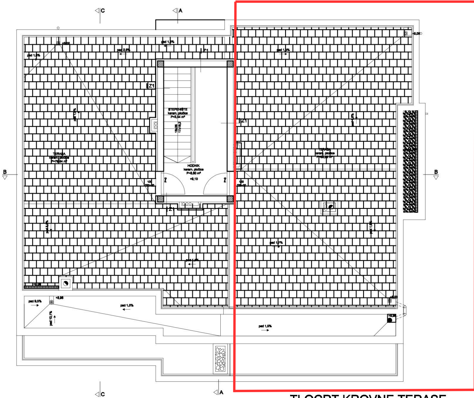
TLOCRT KROVNE TERASE
