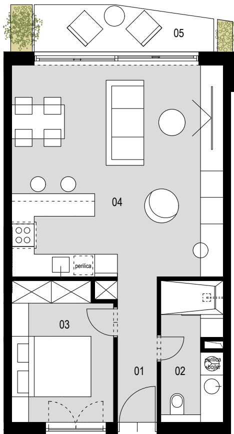
TLOCRT STANA M 1:100 S21
