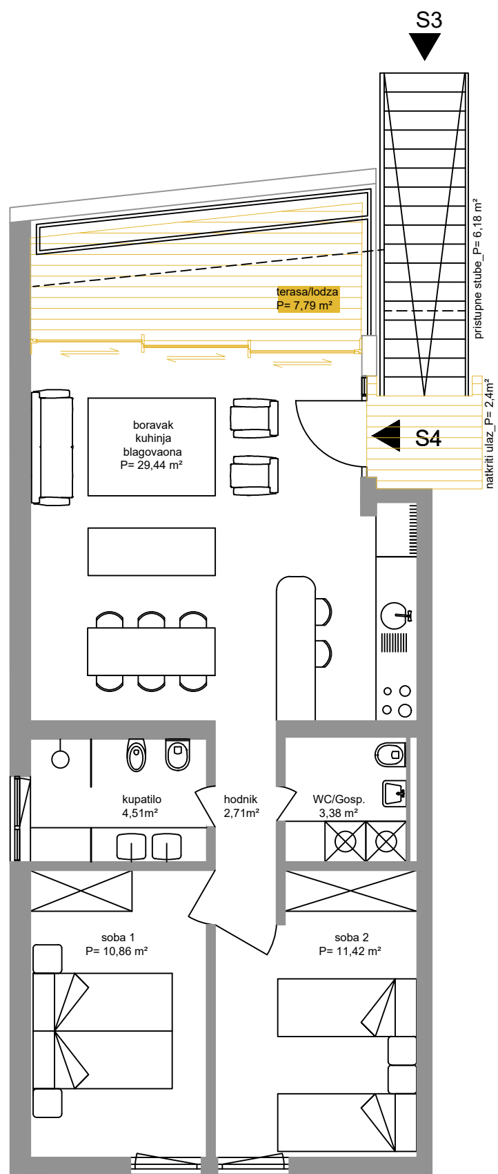
Layout stan S3_visoko prizemlje
