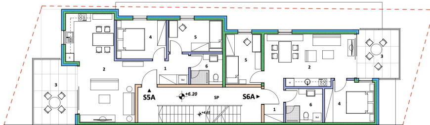
PLANIRANA SUSJEDNA POLUUGRAĐENA VIŠESTAMBENA GRAĐEVINA "B" SA ŠEST (6) STAMBENIH JEDINICA - PO PRIJEDLOGU PARCELAČIJE
