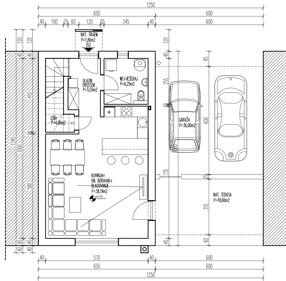
TLOCRT PRIZEMLJA
