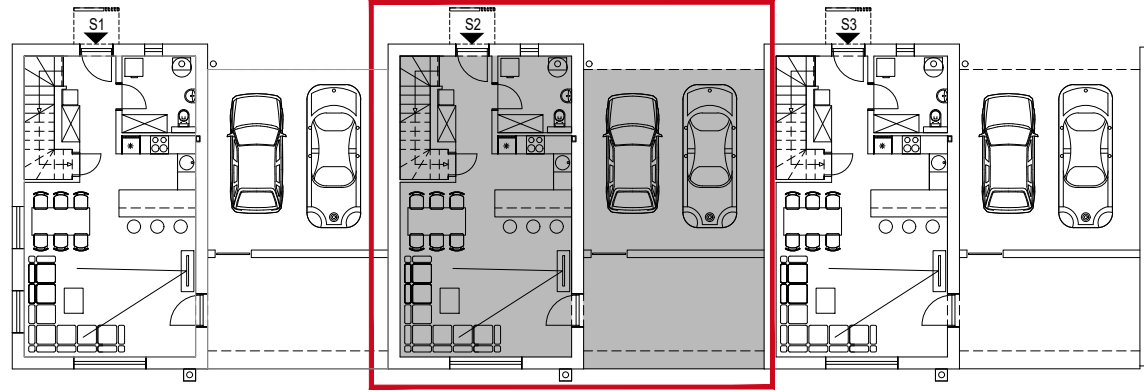
TLOCRT PRIZEMLJA
