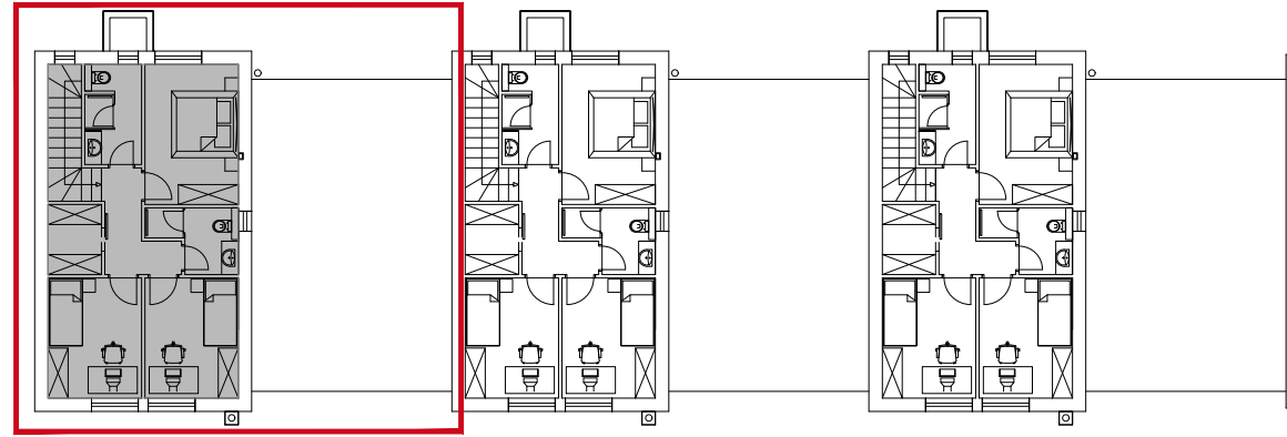
TLOCRT KATA
