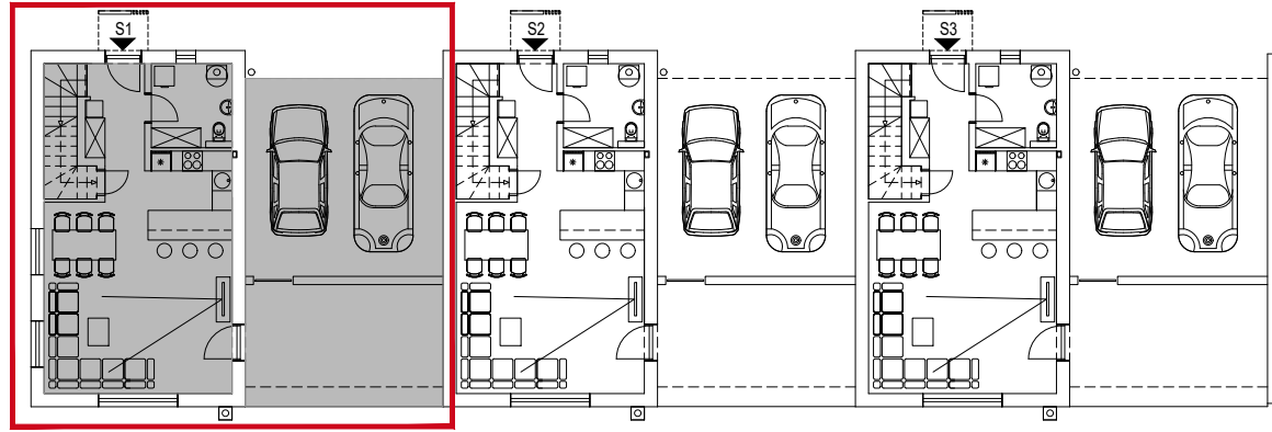
TLOCRT PRIZEMLJA
