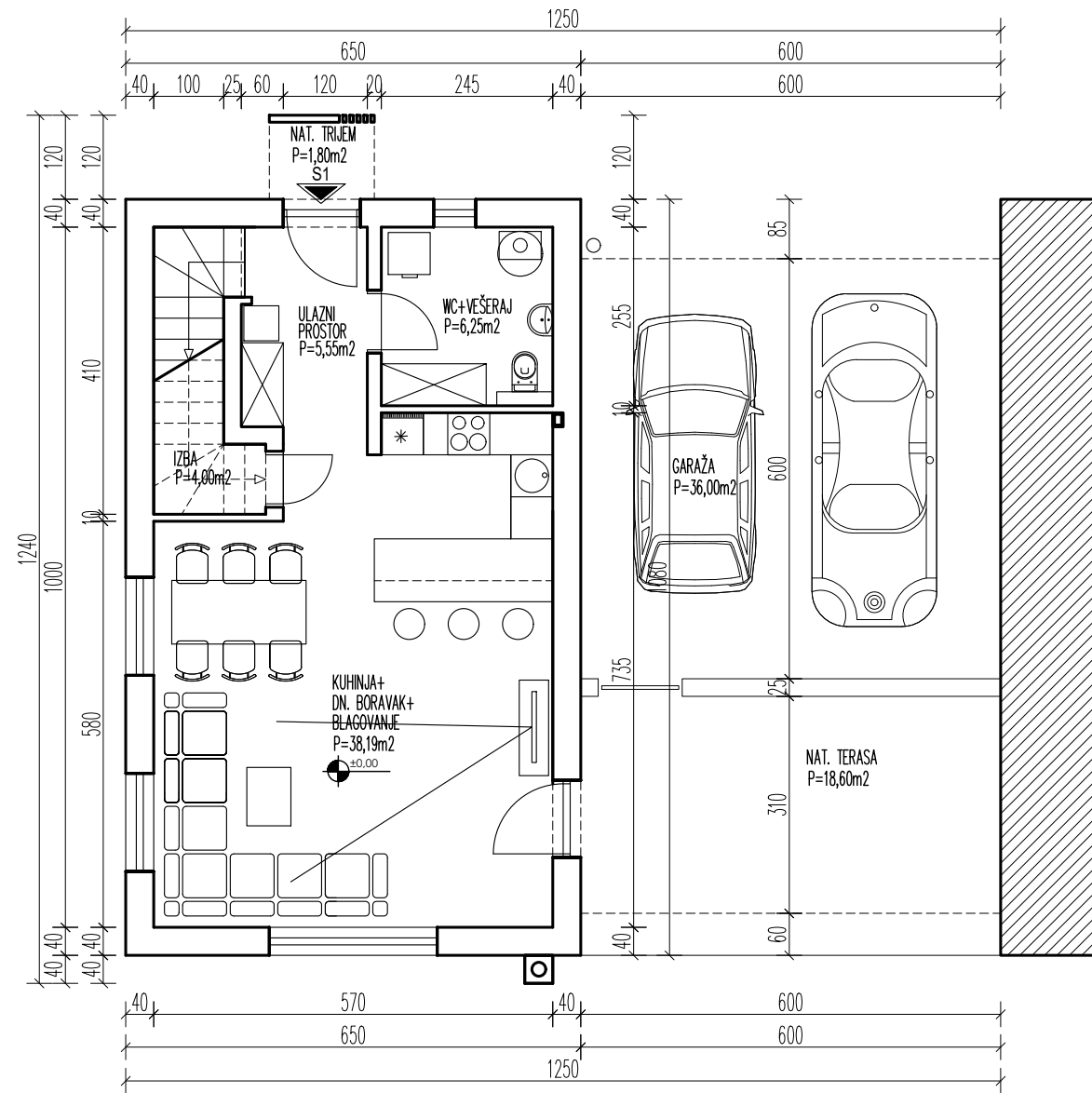
TLOCRT PRIZEMLJA
