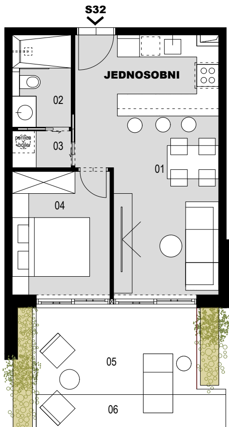
TLOCRT STANA M 1:100
