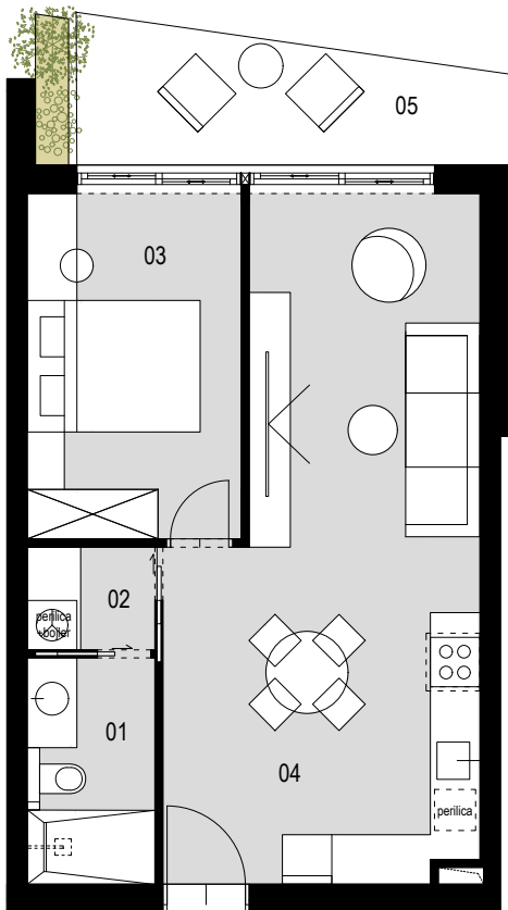
S35 TLOCRT STANA M 1:100
