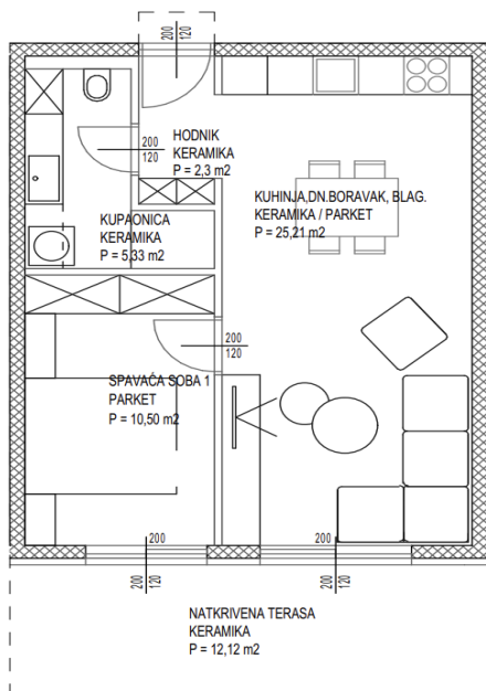
Tlocrt stana
