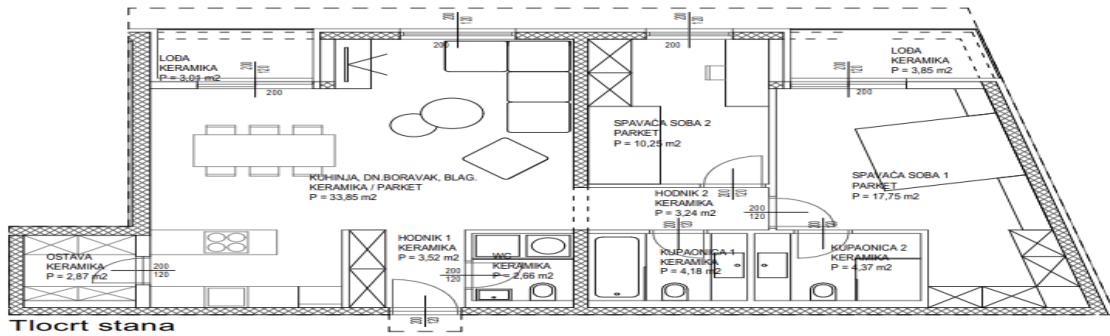
Tlocrt stana
